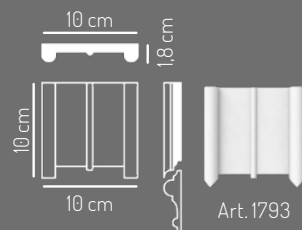
Terminale per Art. 2163
