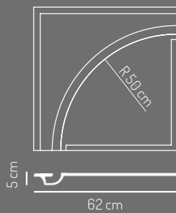
Art. 1803 Parte elettrica non inclusa
