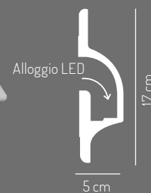
Art. 1801 Parte elettrica non inclusa
