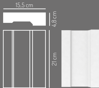
Art. 1829 Zoccolo per Art. 2386
