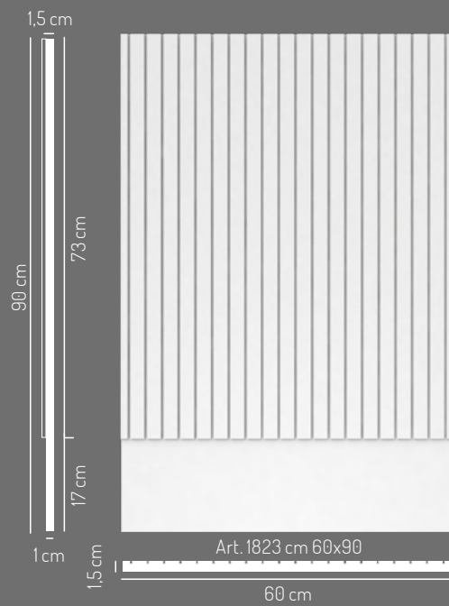
Composizione con: Battiscopa Art. 2395 - Pannello Art.1823 - Marcapiano Art.2389 - Cornice Art. 2253
