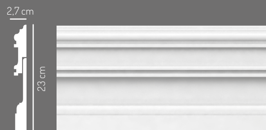
*Esempio per ingombro con minima altezza, 23 cm
