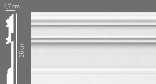
*Esempio per ingombro con massima altezza, 26 cm
